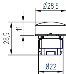
Масса – 0,016 кг Рисунок А.3 – Головка сигнальной лампы OptiSignal D22 C4-L
