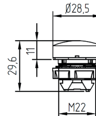
Масса – 0,009 кг Рисунок А.4 – Головка сигнальной лампы OptiSignal D22 C5-L
