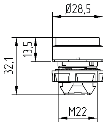
Масса – 0,012 кг Рисунок А.15 – Головка кнопки с выступающим толкателем OptiSignal D22 C5-PJ
