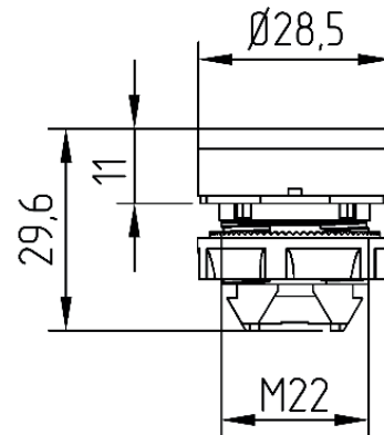
Масса – 0,012 кг Рисунок А.16 – Головка кнопки с подсветкой OptiSignal D22 C5-PL
