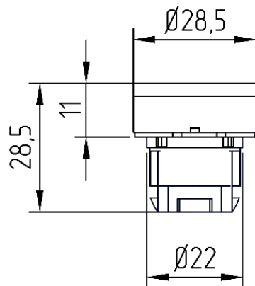
Рисунок А.13 – Головка кнопки с подсветкой OptiSignal D22 C4-PL
