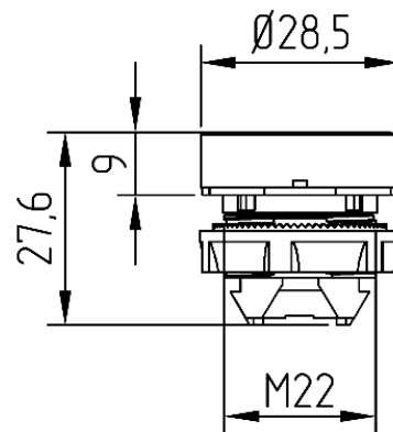
Рисунок А.12 – Головка кнопки с выступающим толкателем OptiSignal D22 C4-PJ
