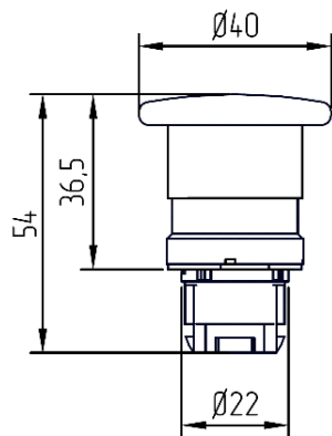
Масса – 0,06 кг Рисунок А.17 – Головка кнопки аварийного останова, возврат поворотом OptiSignal D22 A4-ESTR
