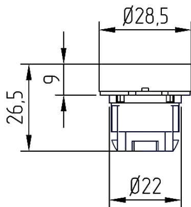
Рисунок А.11 – Головка кнопки OptiSignal D22 C4-P
