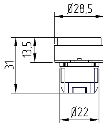
Рисунок А.12 – Головка кнопки с выступающим толкателем OptiSignal D22 C4-PJ
