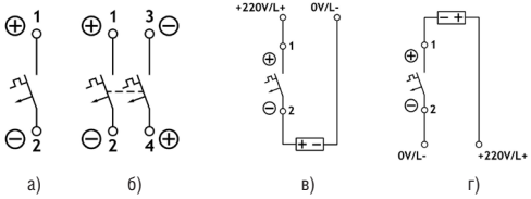
Рисунок Г.1 - Принципиальные электрические схемы выключателей
