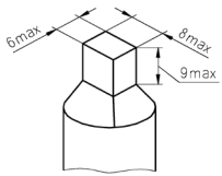
Рисунок Д.1 - Форма и размеры проводника, подготовленного для присоединения к выключателю
