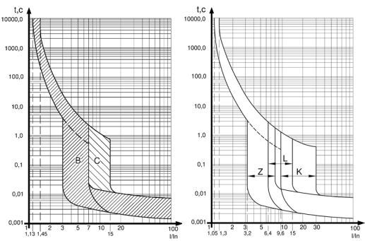
Рисунок Б.3 - Защитные характеристики В, С в цепи постоянного тока при контрольной температуре плюс 30 °С Рисунок Б.4 - Защитные характеристики Z, L, K в цепи постоянного тока при контрольной температуре плюс 30 °С
