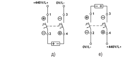
а) однополюсного; б) двухполюсного и примеры подключения в сетях постоянного тока в), г) однополюсного; д), е) двухполюсного
