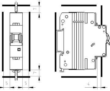
Рисунок Е.1 - Минимально допустимые расстояния от выключателя до металлических частей распределительного устройства Гибкие проводники должны быть изолированы на длине не менее 20 мм от выключателя.
