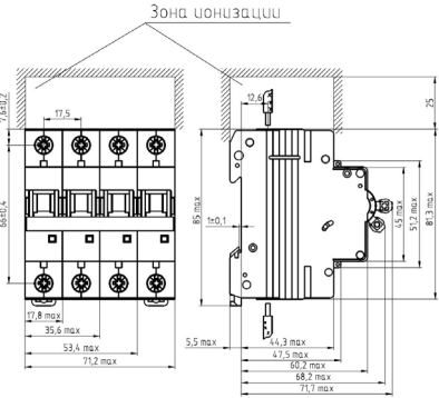
Рисунок В.1 - Габаритные и установочные размеры выключателей
