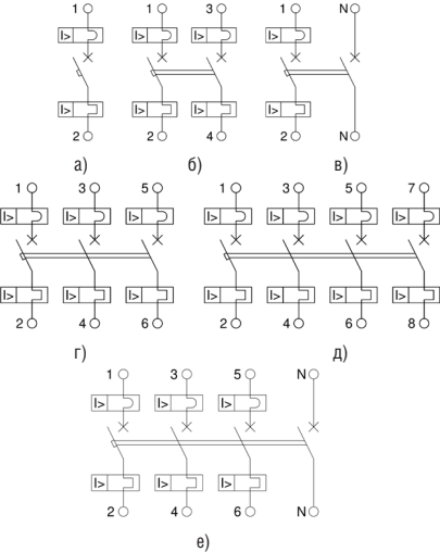
а) однополюсного; б) двухполюсного с двумя защищенными полюсами; в) двухполюсного с одним защищенным и нейтральным полюсами; г) трёхполюсного; д) четырёхполюсного с четырьмя защищенными полюсами; е) четырёхполюсного с тремя защищенными полюсами.
