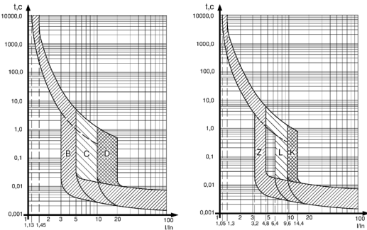
Рисунок Б.1 - Защитные характеристики В, С, D в цепи переменного тока при контрольной температуре плюс 30 °С Рисунок Б.2 - Защитные характеристики Z, L, K в цепи переменного тока при контрольной температуре плюс 30 °С
